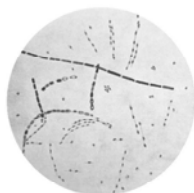
Antraks bakterija
